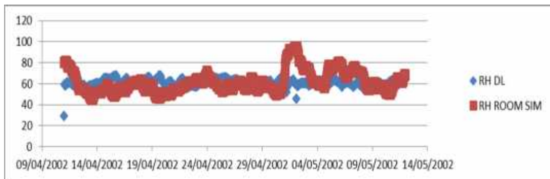
شکل ۱۱. بررسی مقایسه‌ای نمودارهای اطلاعات رطوبت نسبی بازه یک ماهه توسط دیزاین بیلدر و دیتالاگر
