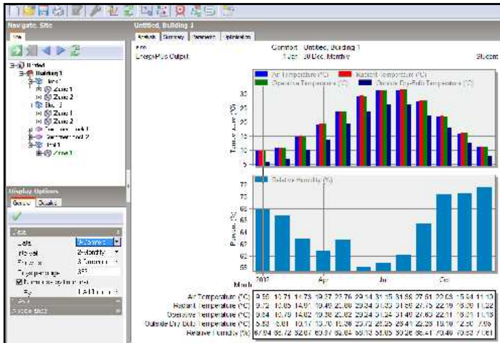
شکل ۸. اطلاعات اقلیمی دما و رطوبت ماهانه در محدوده اسایش اتاق اصلی زندگی ساکنین در ساختمان پروژه باتحلیل نرم افزار دیزاین بیلدر
